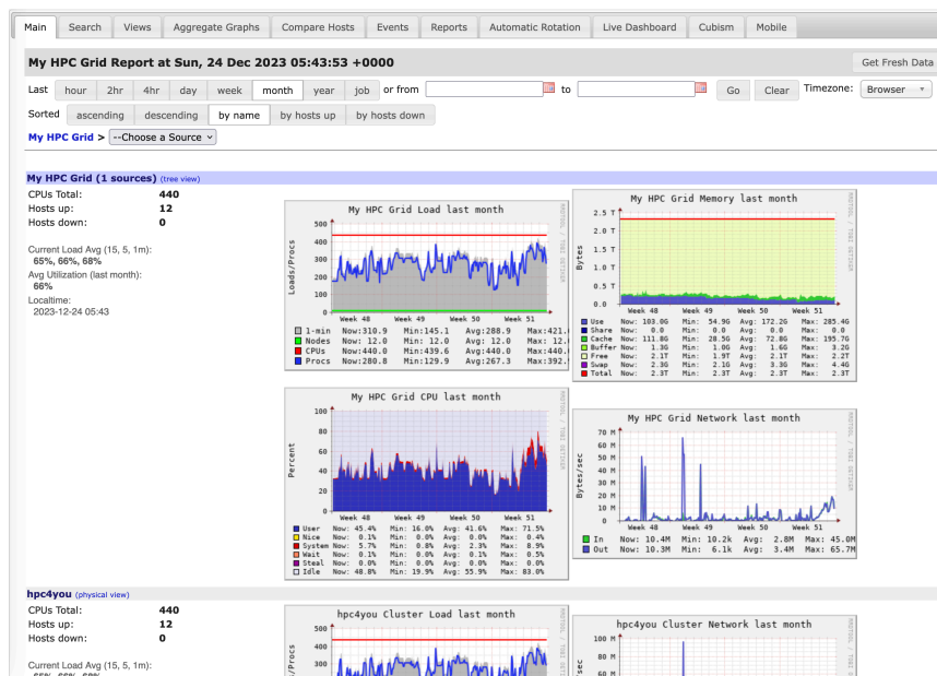
图 17: Ganglia集群性能监测示例。
